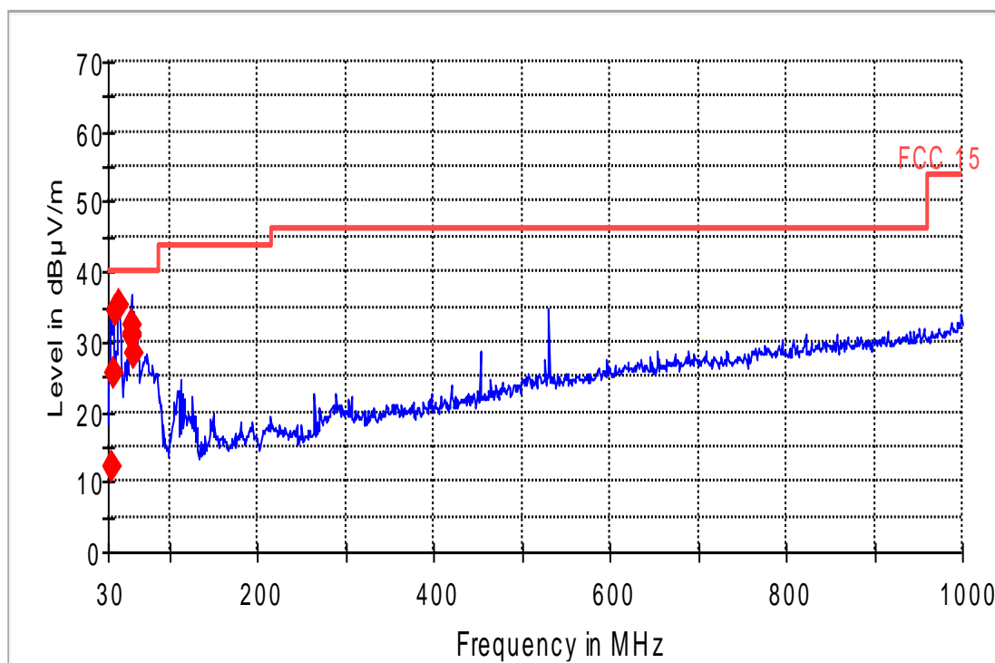
FCC 15 30-1000MHz
