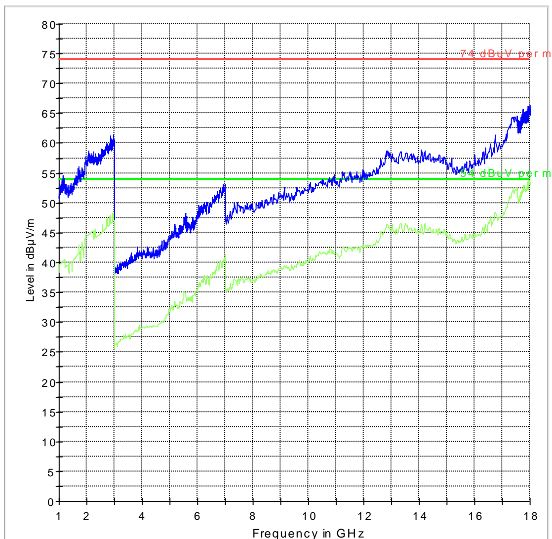
FCC 15 1-18GHz
