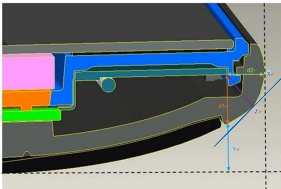
WWAN Antenna: X=00mm, Y=4.03mm, Z=3.76mm, d1=3.42mm, d2=2.77mm
