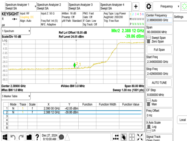
802.11g_20MHz_Chain1_2427MHz
