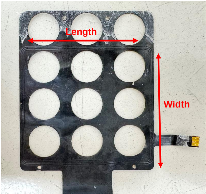
FPCB Antenna(YMM624)
