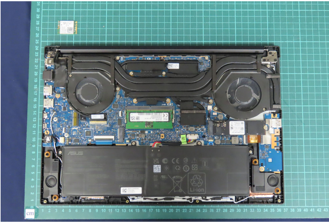
(18) EUT Photo
