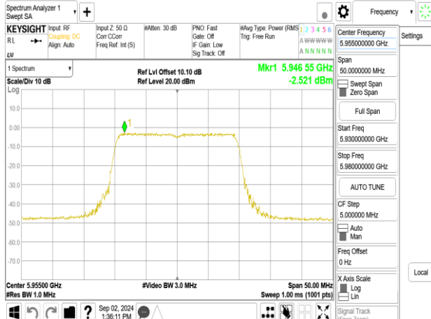
802.11be_20MHz_Chain0_5955MHz
