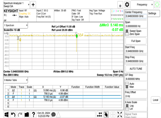
802.11be_20MHz_Chain0_5955MHz_RU52_37
