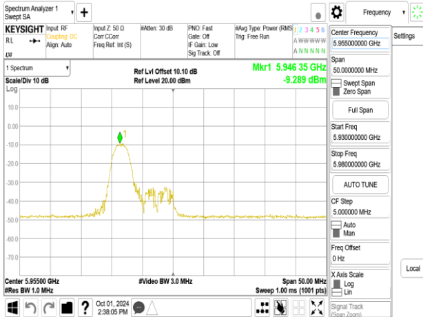
802.11be_20MHz_Chain0_5955MHz_RU52_37
