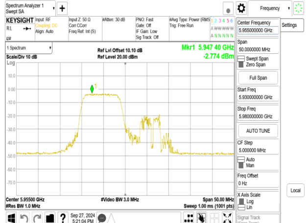
802.11be_20MHz_Chain0_5955MHz_RU106_53
