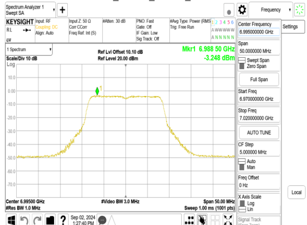
802.11a_20MHz_Chain0_6995MHz
