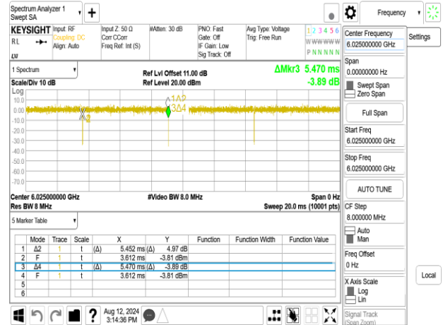
802.11be_160MHz_Chain0_6025MHz_996+484_MRU4
