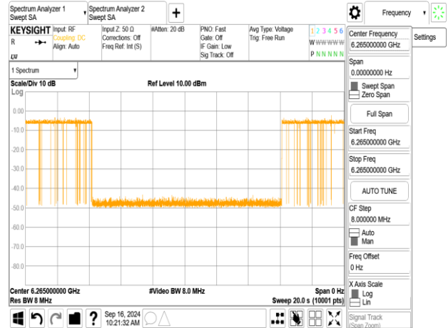
802.11be_320MHz_CF 6265MHz_Interference_6110MHz_-77.93dBm_Minimal 802.11be_320MHz_CF 6265MHz_Interference_6265MHz_-76.9dBm_Minimal
