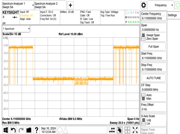
802.11be_320MHz_CF 6265MHz_Interference_6110MHz_-77.93dBm_Minimal 802.11be_320MHz_CF 6265MHz_Interference_6265MHz_-76.9dBm_Minimal
