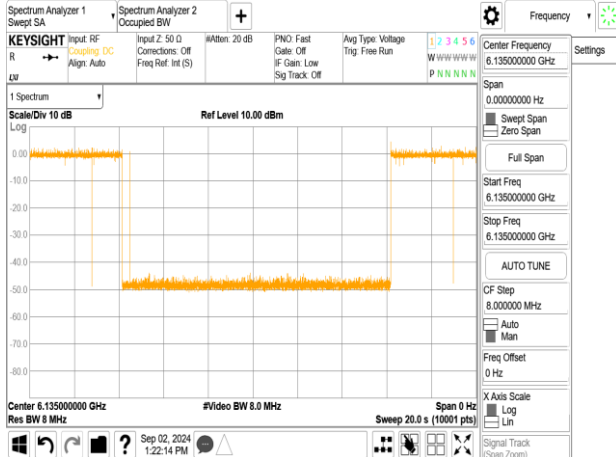
802.11be_20MHz_CF 6135MHz_Interference_6135MHz_-78.86dBm_ON
