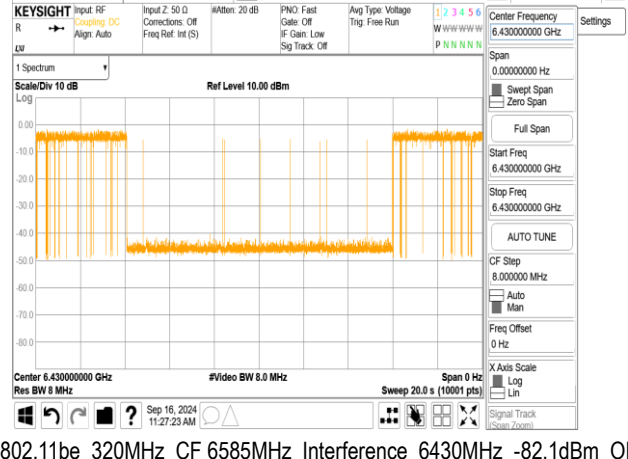
802.11be_320MHz_CF 6585MHz_Interference_6430MHz_-82.1dBm_ON
