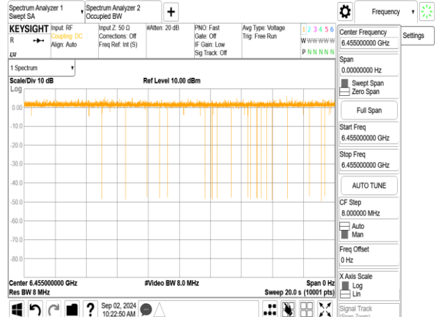
802.11be_20MHz_CF 6455MHz_Interference_6455MHz_-76.99dBm_ON
