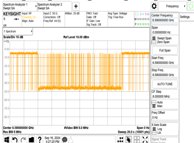
802.11be_320MHz_CF 6745MHz_Interference_6590MHz_-80.05dBm_ON
