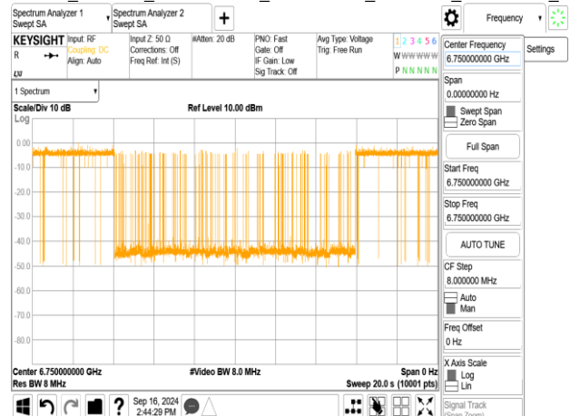
802.11be_320MHz_CF 6905MHz_Interference_6750MHz_-80.69dBm_ON
