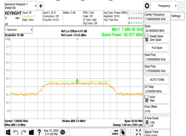
802.11be_320MHz_6905MHz_AWGN:7060MHz
