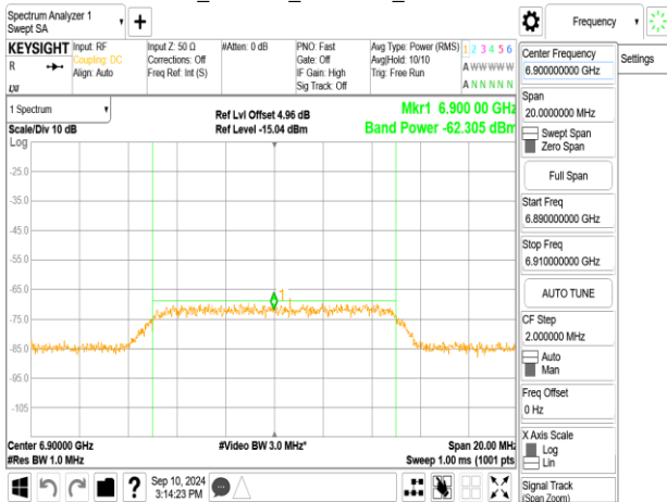
802.11be_320MHz_6905MHz_AWGN:6750MHz
