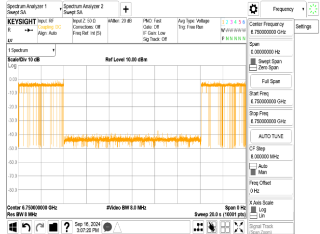
802.11be_320MHz_CF 6905MHz_Interference_6750MHz_-77.69dBm_Minimal
