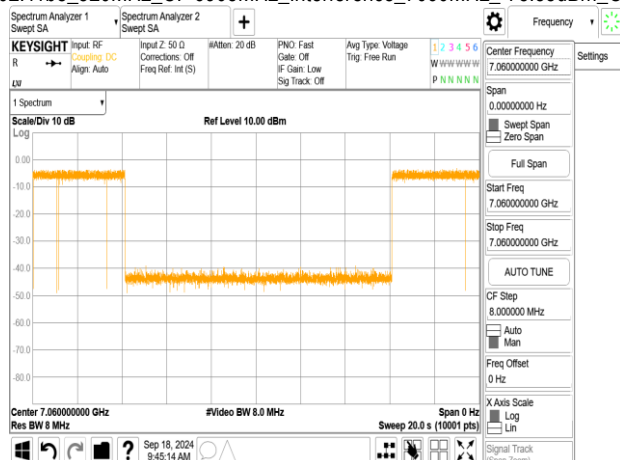
802.11be_320MHz_CF 6905MHz_Interference_7060MHz_-79.55dBm_Minimal
