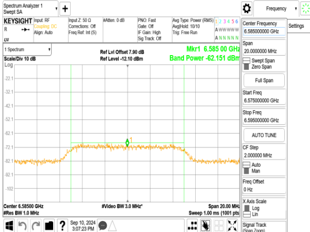
802.11be_320MHz_6585MHz_AWGN:6585MHz
