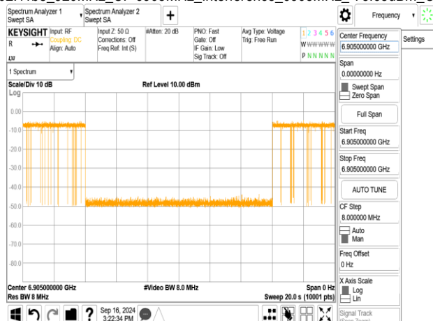
802.11be_320MHz_CF 6905MHz_Interference_6905MHz_-76.65dBm_Minimal
