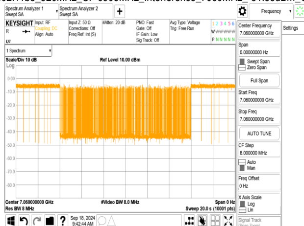
802.11be_320MHz_CF 6905MHz_Interference_7060MHz_-81.55dBm_ON
