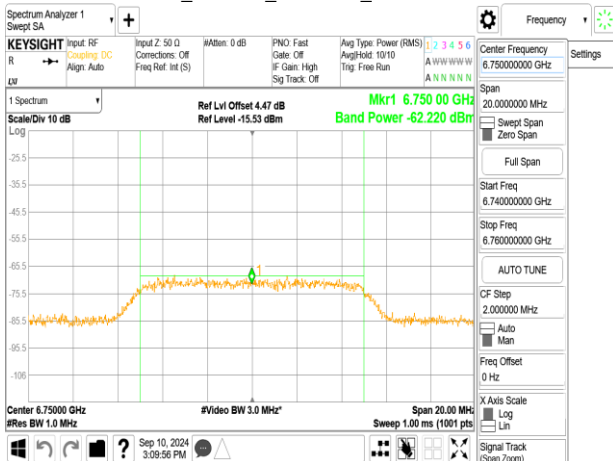
802.11be_320MHz_6905MHz_AWGN:6750MHz
