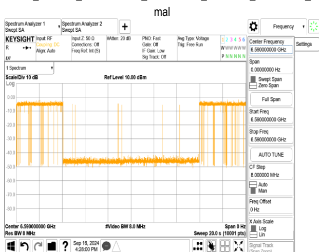
802.11be_320MHz_CF 6745MHz_Interference_6590MHz_-80.05dBm_ON
