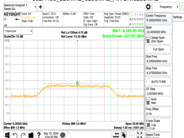
802.11be_320MHz_6265MHz_AWGN:6265MHz
