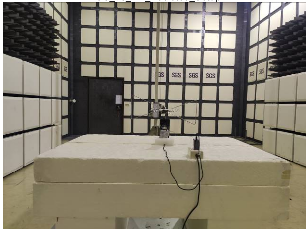
FCC_15_407_WLAN_6E_Normal_CBP_Setup
