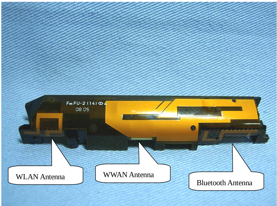
(20) EUT Photo
