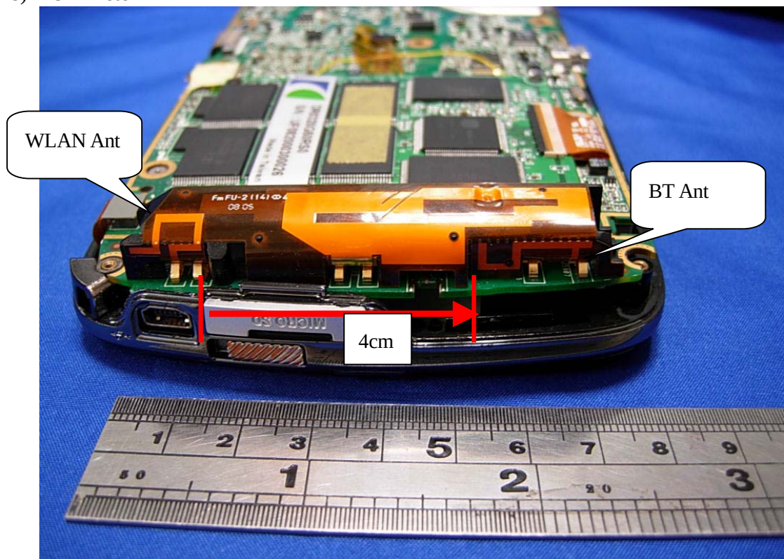
(18) EUT Photo
