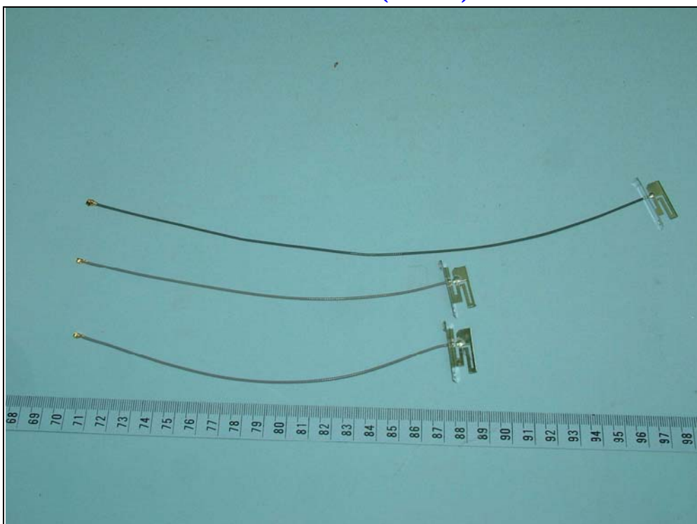
Laird antenna (3.97dBi)
