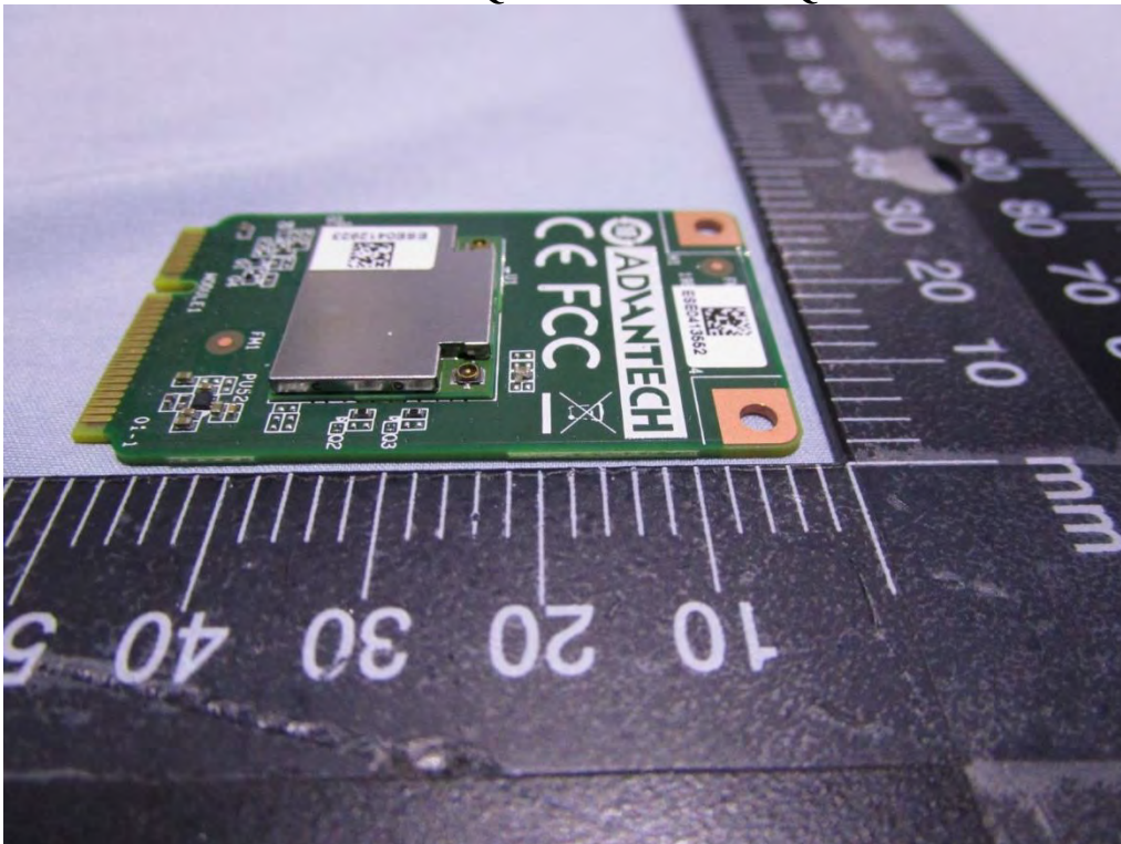
Outview: AIW-173HQ-GI1 & AIW-173HQ-GI2 Pic 6
