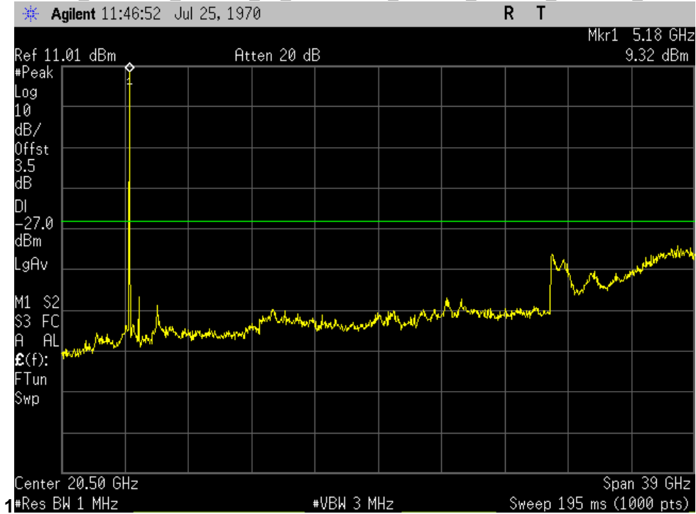
U-NII-1_5180MHz_Low_Ch_36_20MHz_BW_a-mode_-27dBm_1-40GHz_Port
