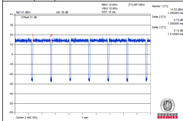
802.11n (HT20)
