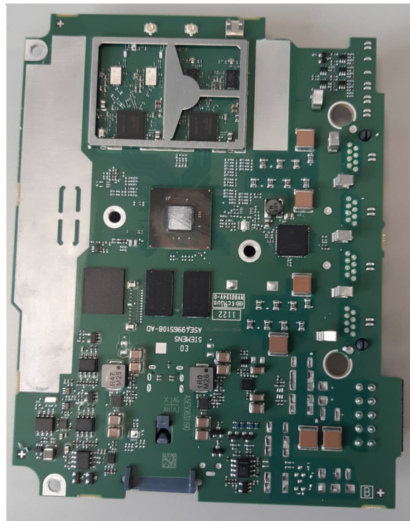
MSAX-W1-RJ-E2-NO
