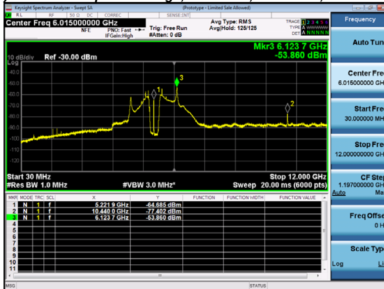
Antenna A
