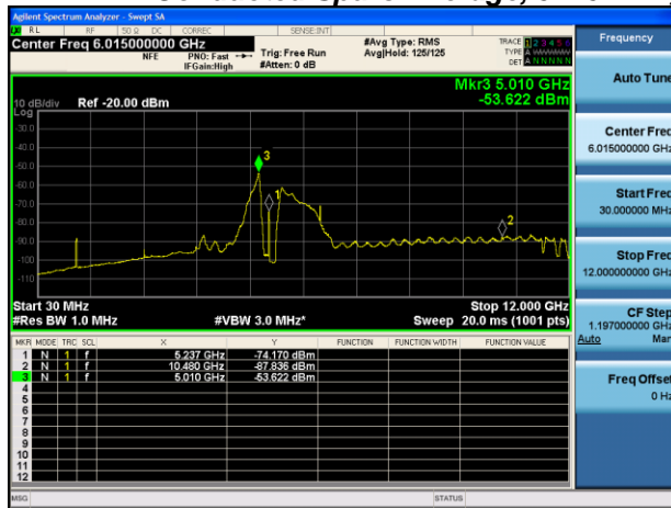
Antenna A
