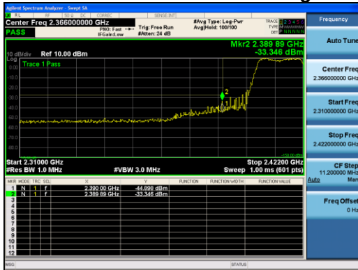
Antenna A
