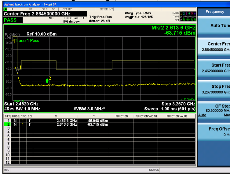
Antenna A
