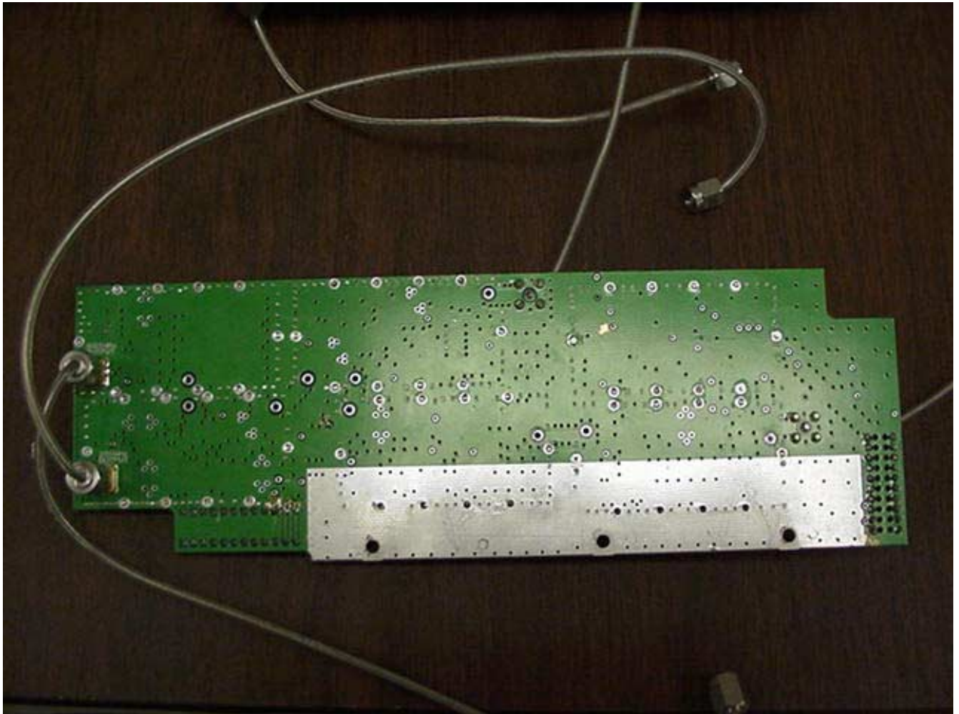
LO GEN Board Bottom Side
