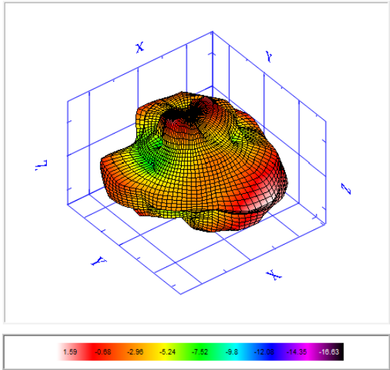
2500MHZ
