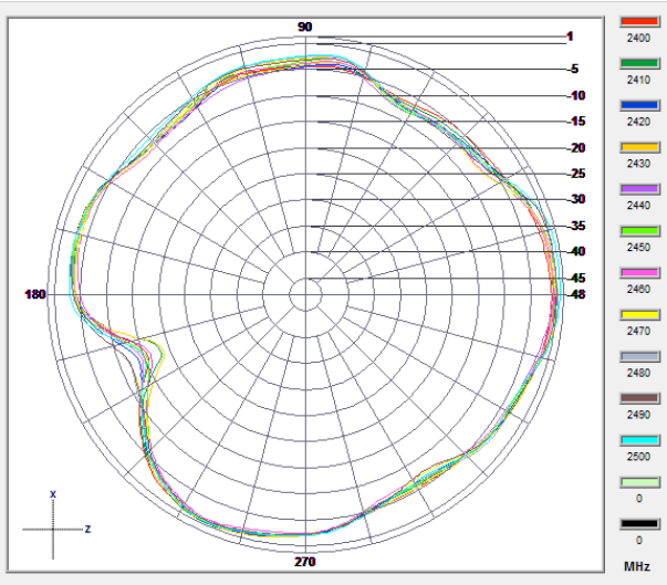
XZ
