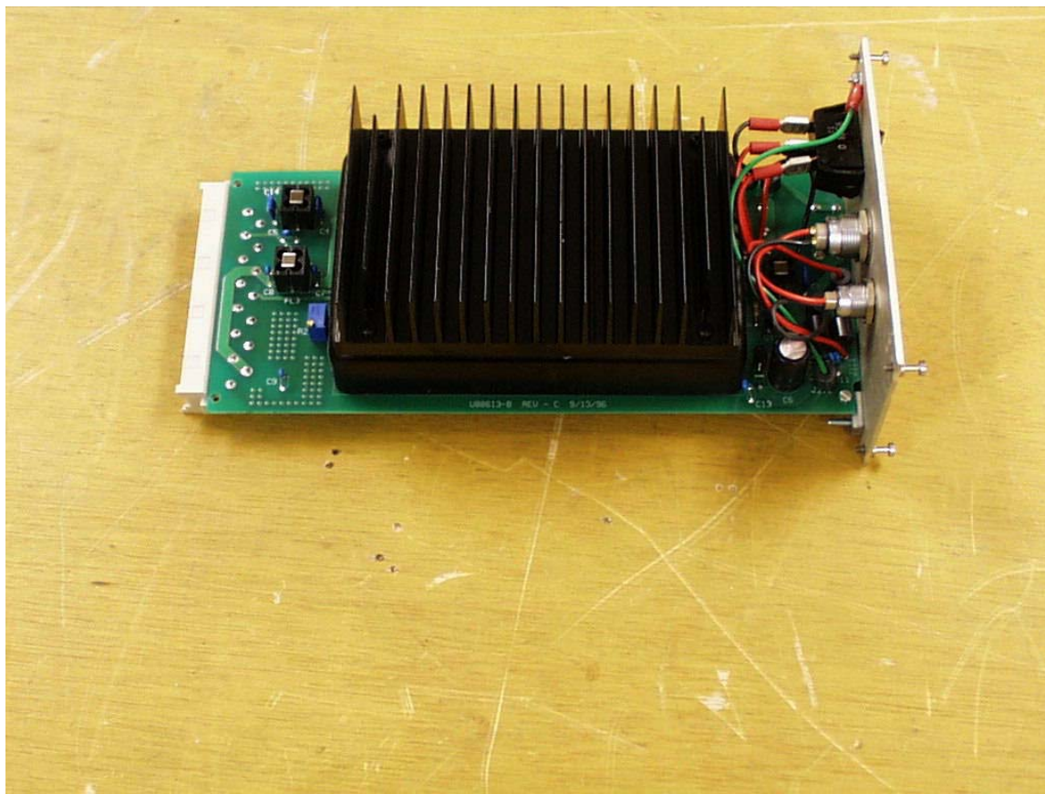
Power input module top
