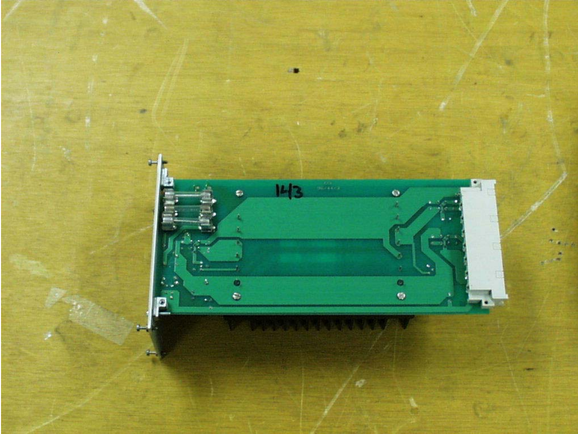
Power input module bottom
