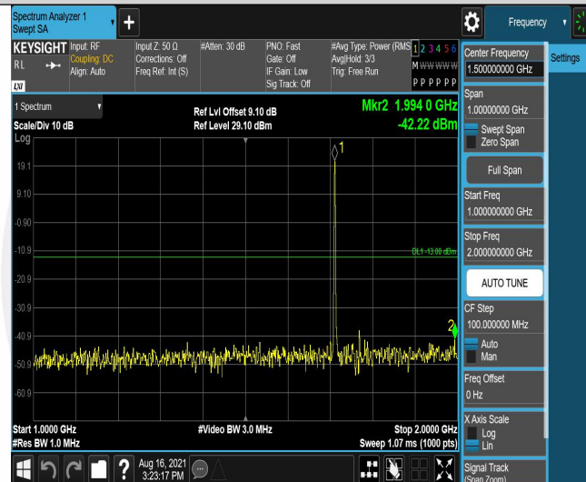
Band4-1.4MHz-16QAM-19957-6RB#0-Range2:1000~2000MHz
