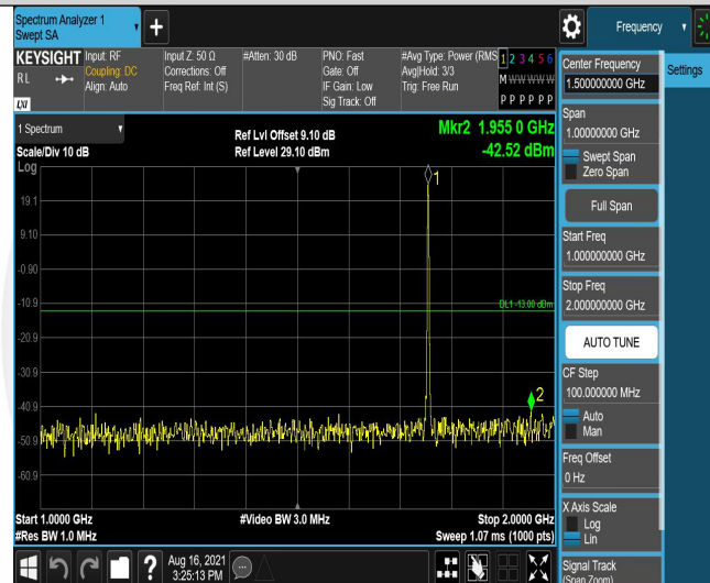
Band4-1.4MHz-QPSK-20393-6RB#0-Range2:1000~2000MHz
