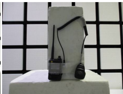
Z-plane
