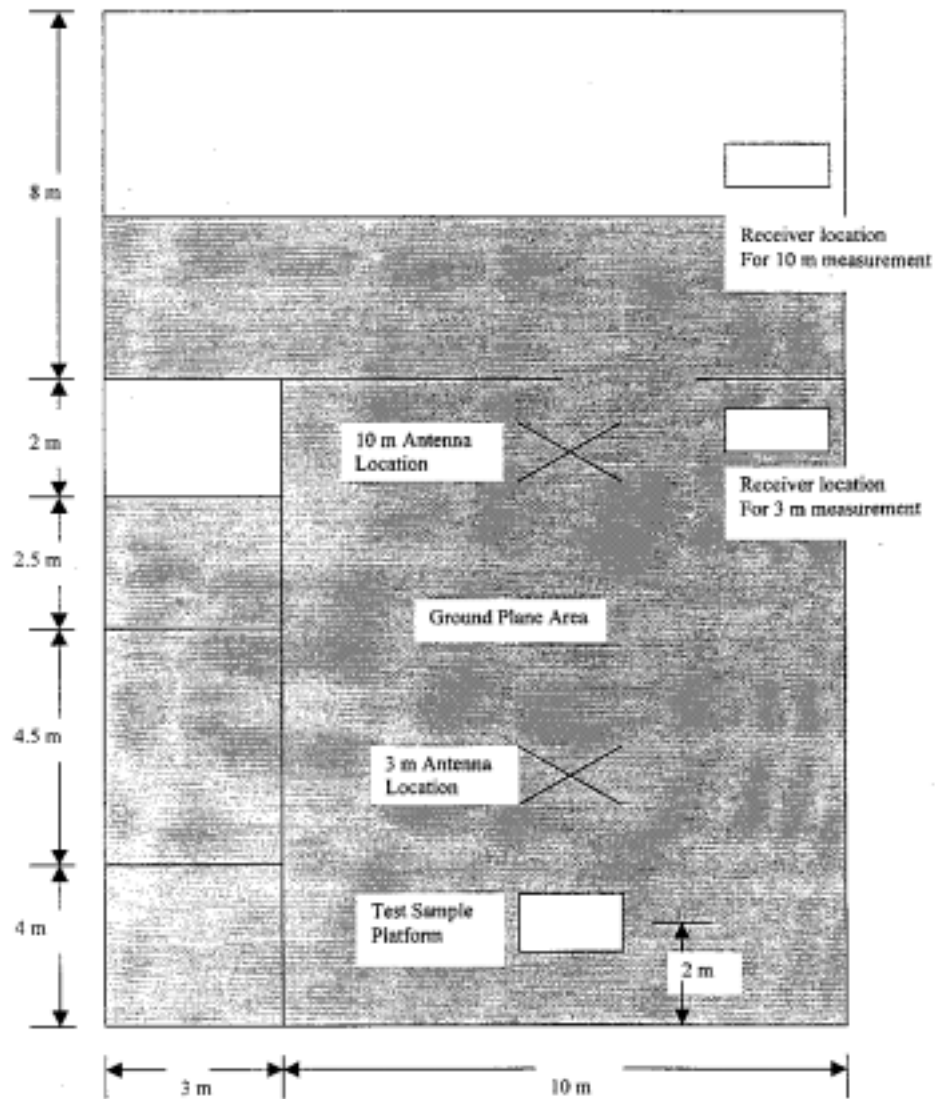
OATS TEST SITE LAYOUT
