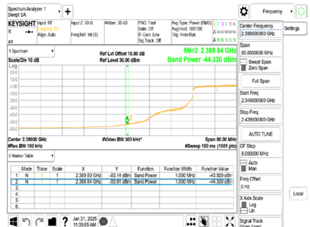
SISO_802.11n_20MHz_Chain0_2427MHz
