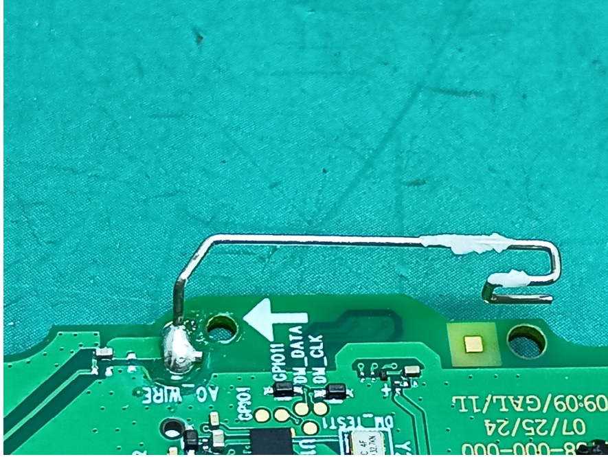
DECT ANT0
