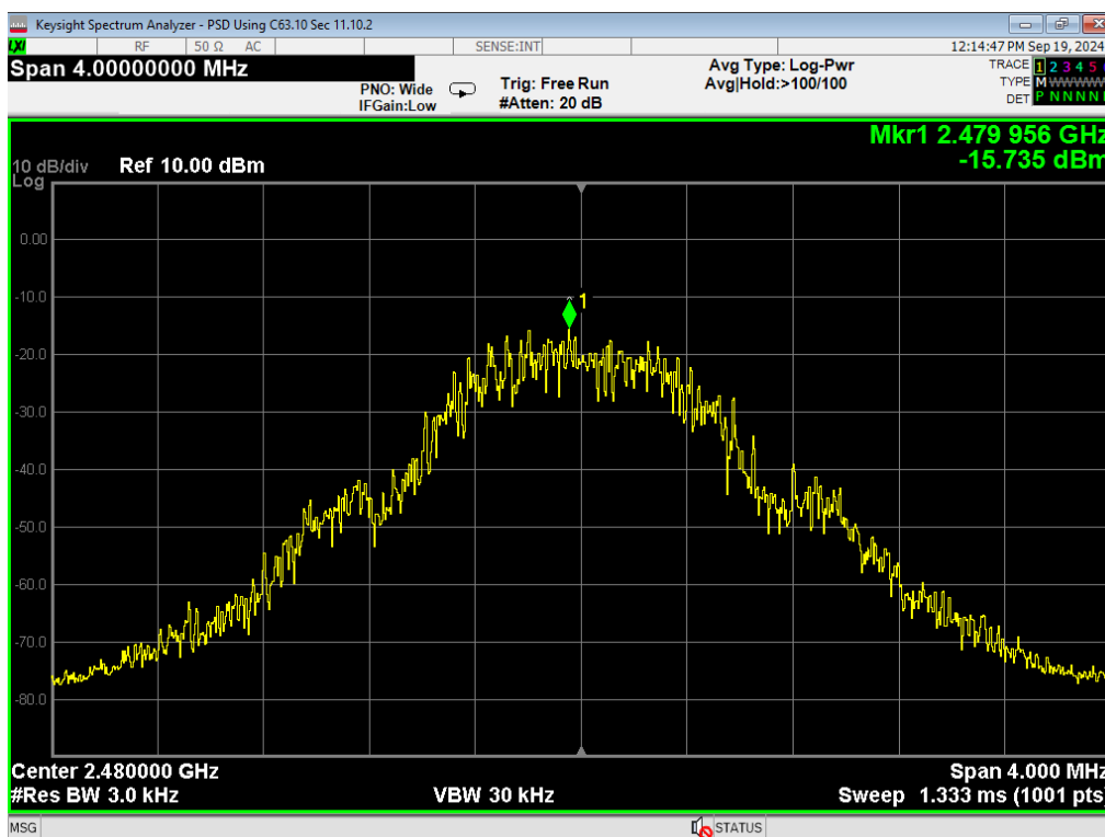
28, PSD, BLE 1MB, High
