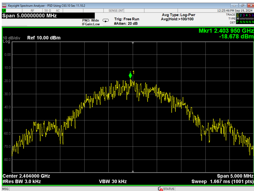
42, PSD, BLE 2MB, Low
