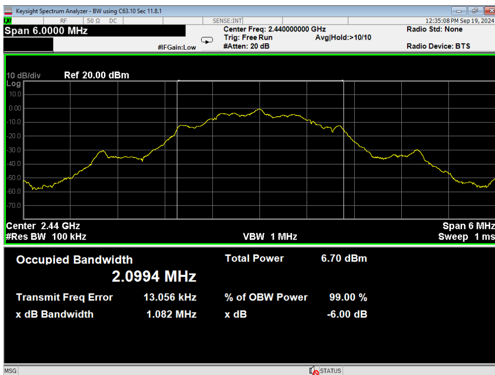
40, 6dB Bandwidth, BLE 2MB, Mid
