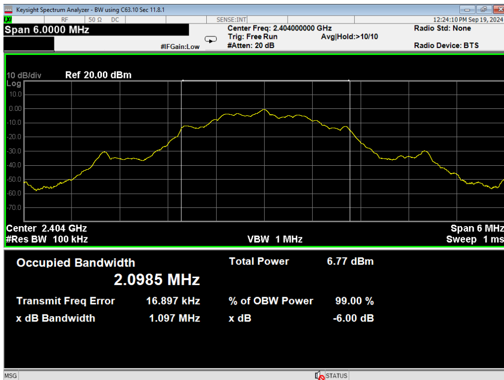
39, 6dB Bandwidth, BLE 2MB, Low
