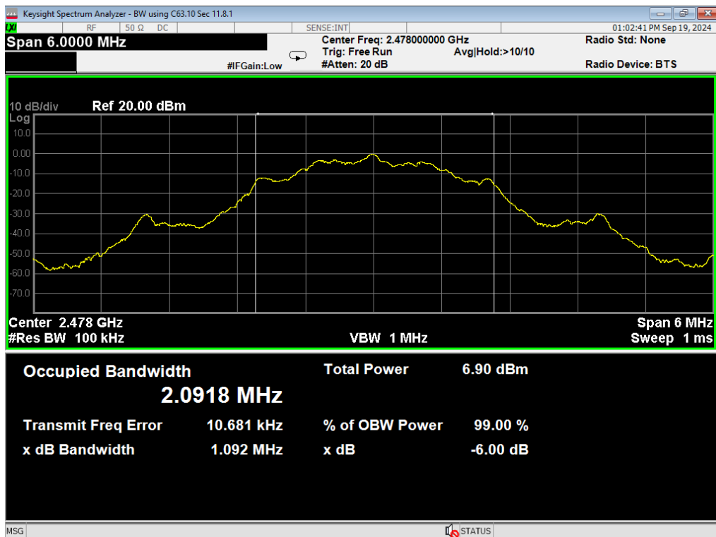
41, 6dB Bandwidth, BLE 2MB, High
