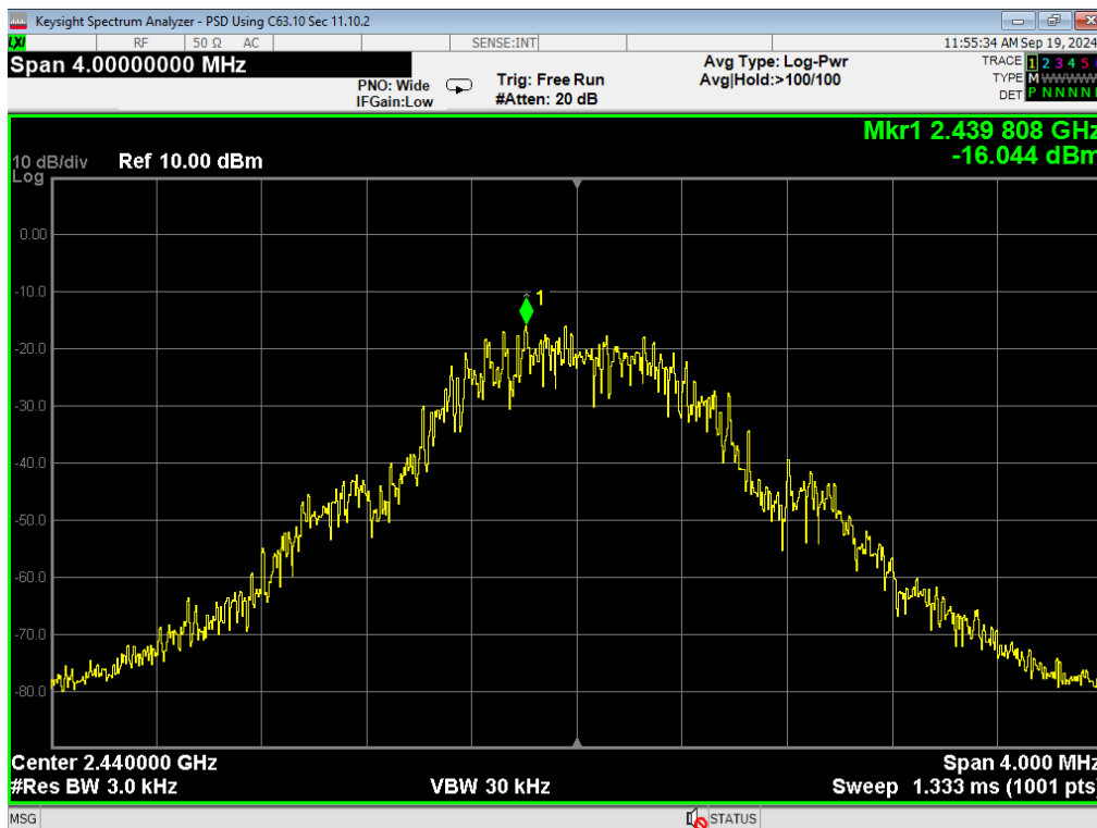
27, PSD, BLE 1MB, Mid
