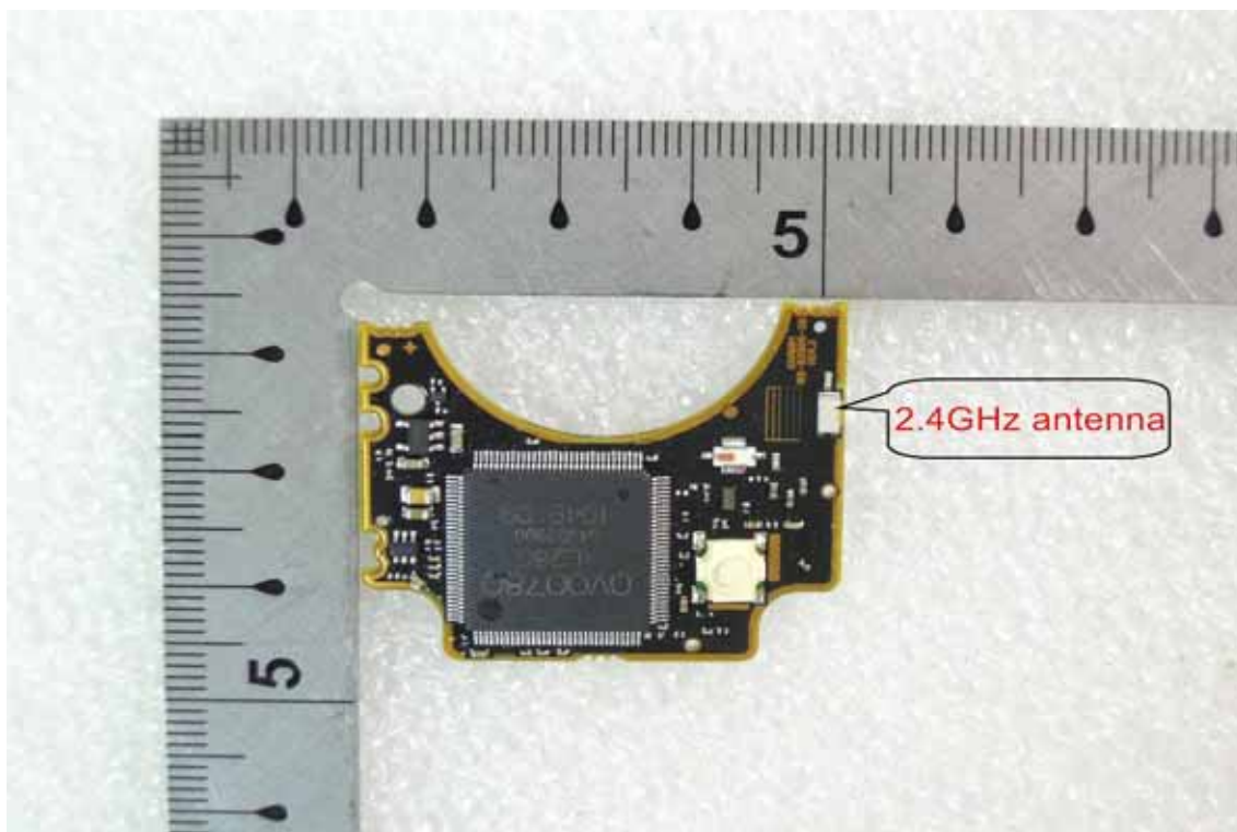
2.4GHz Antenna
