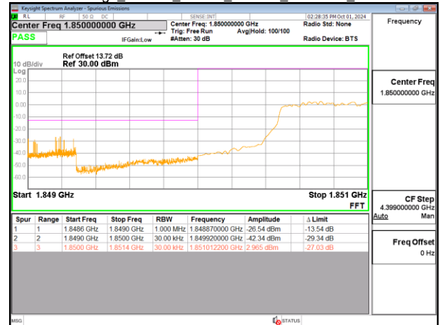
Band Edge_Band25_10MHz_PUSCH_1855MHz_Chain0
