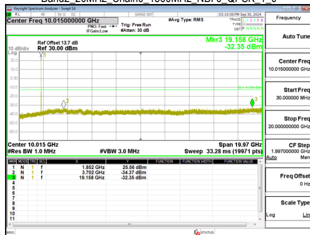
Band2_20MHz_Chain0_1880MHz_NBI 0_QPSK_1_0
