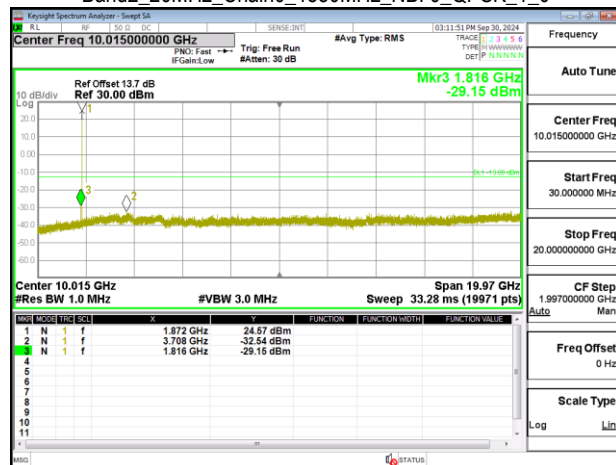
Band2_20MHz_Chain0_1900MHz_NBI 0_QPSK_1_0
