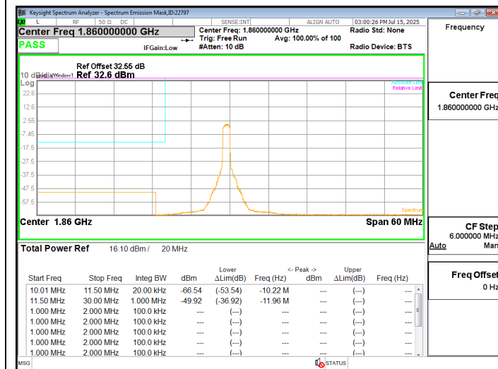
LTE2 20MHz QPSK LOW Ch RB6-0
