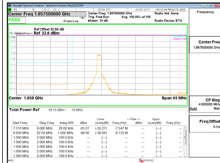
LTE2 15MHz QPSK LOW Ch RB6-0
