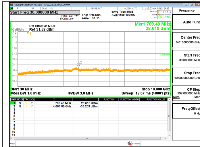
LTE12 5MHz QPSK LOW Ch RB1-0
