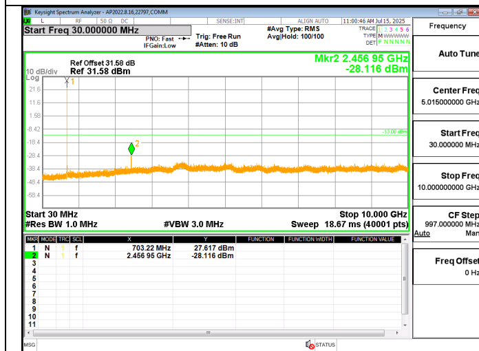
LTE12 10MHz QPSK MID Ch RB1-0
