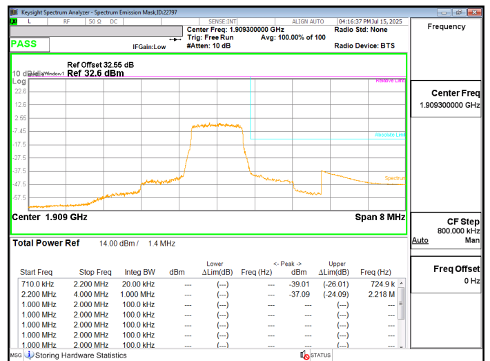
LTE2 1.4MHz QPSK HIGH Ch RB6-0
