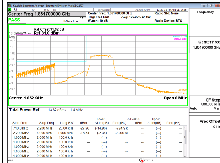
LTE2 1.4MHz QPSK LOW Ch RB6-0
