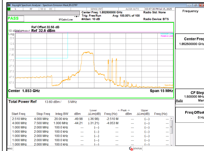
LTE2 5MHz QPSK LOW Ch RB6-0
