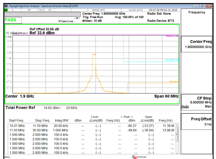
LTE2 20MHz QPSK HIGH Ch RB6-0
