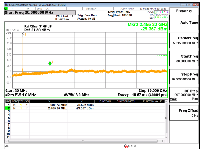
LTE12 10MHz QPSK LOW Ch RB1-0
