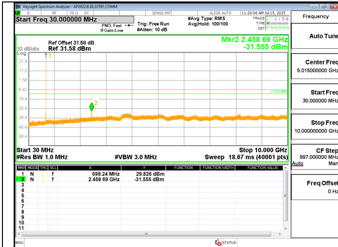
LTE12 1.4MHz QPSK LOW Ch RB1-0
