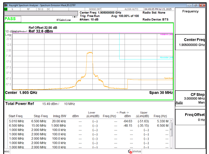
LTE2 10MHz QPSK HIGH Ch RB6-0
