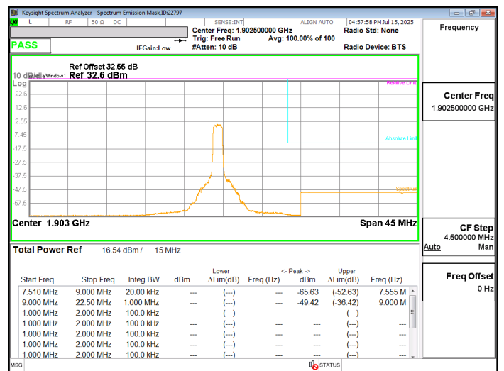
LTE2 15MHz QPSK HIGH Ch RB6-0
