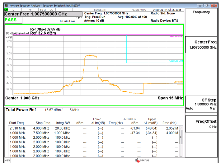
LTE2 5MHz QPSK HIGH Ch RB6-0
