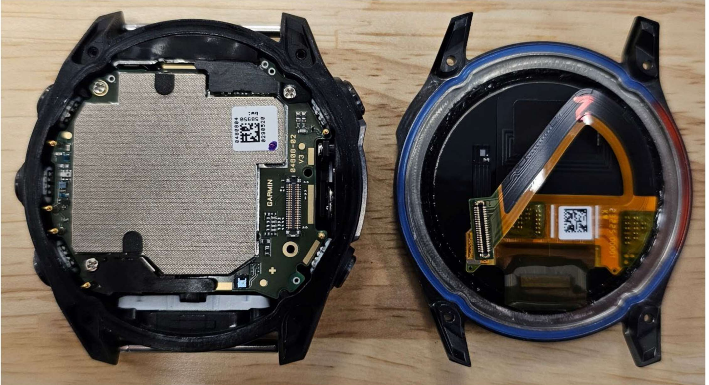
Figure E14.1 – Internal – DUT Split
