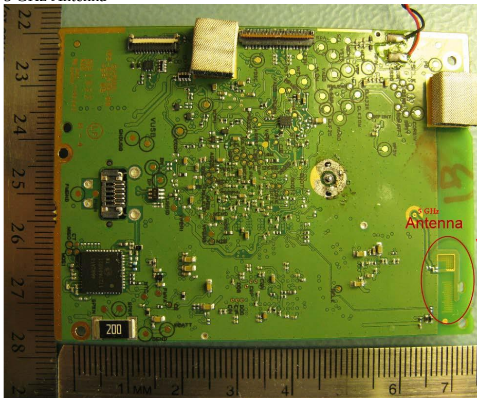
5 GHz Antenna
