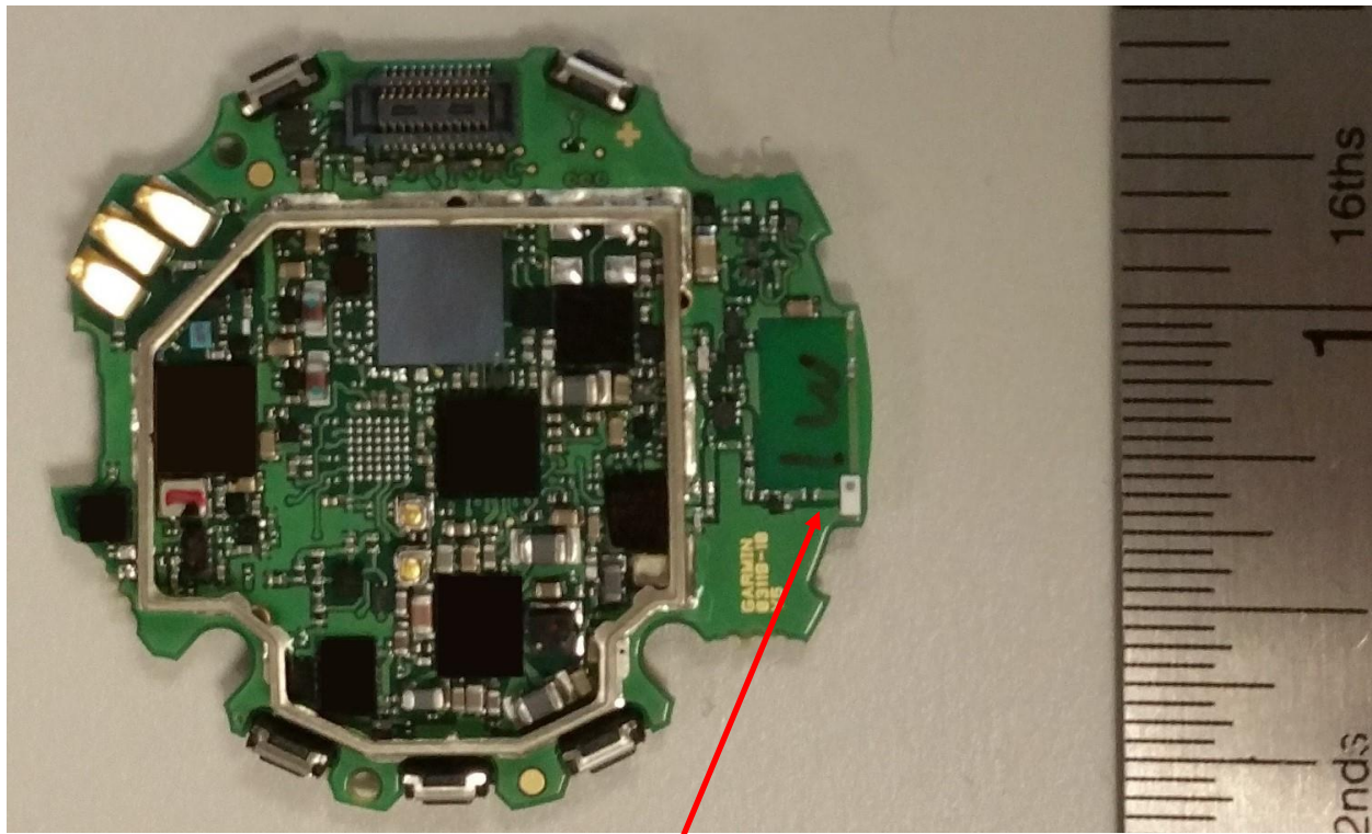
Antenna
