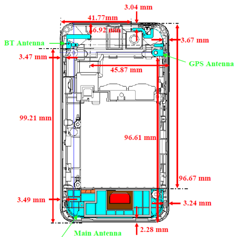
Fig.19 Antenna
