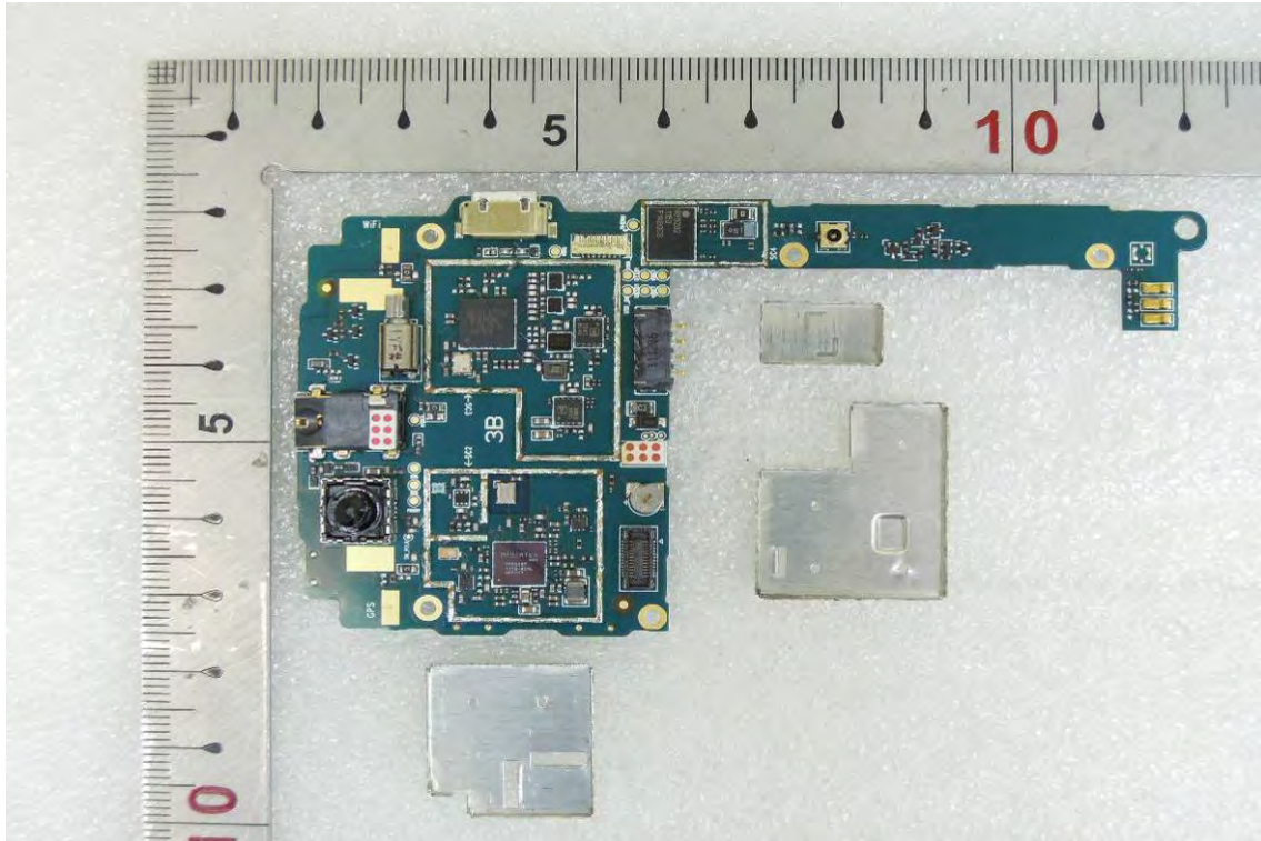
BT/ WLAN & GPS Antenna
