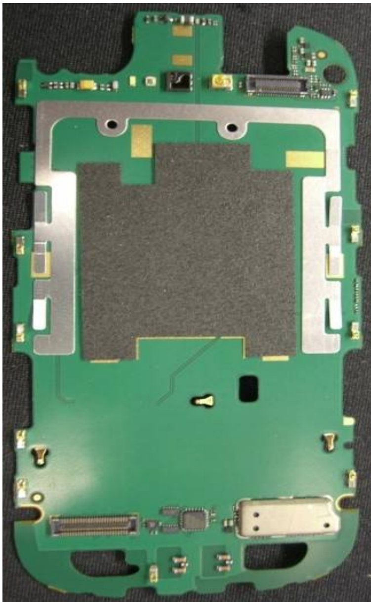
ICB Top Side
