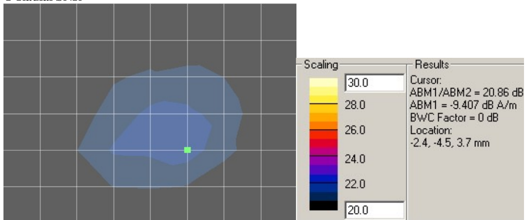
Y Radial SNR
