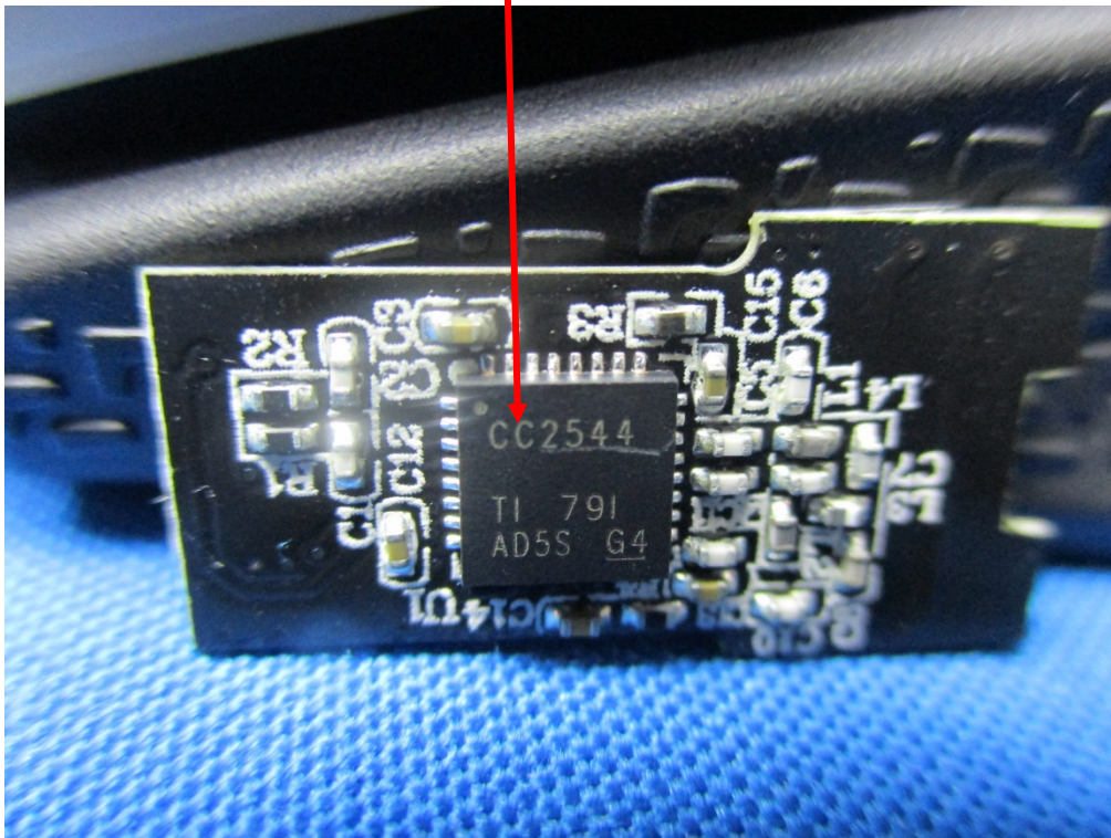
IC – Top View
