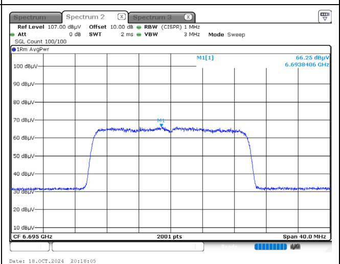
802.11be / 20MHz / 6695MHz / Ch149
