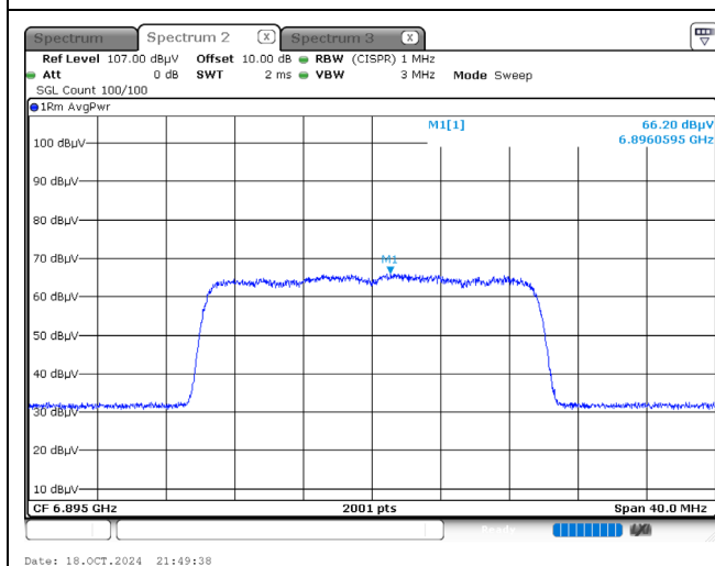
802.11be / 20MHz / 6895MHz / Ch189
