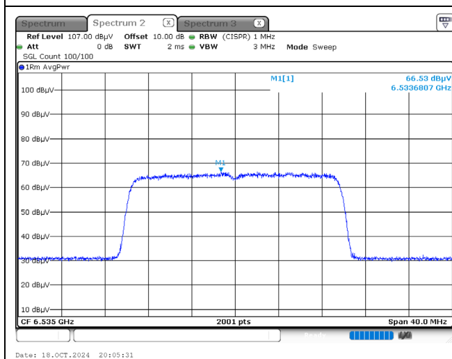
802.11be / 20MHz / 6535MHz / Ch117
