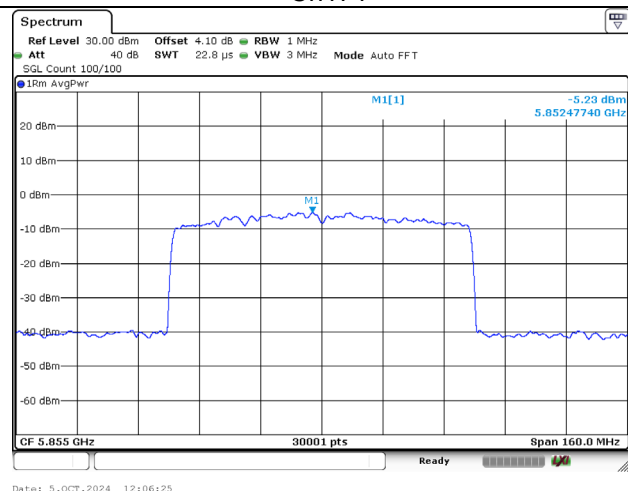
802.11be / 80MHz / Ant.2 / MCS0 / 5855MHz / Ch171
