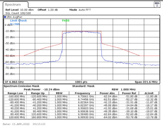
802.11ax (80MHz) / 6865MHz / Chain D / NSS-1
