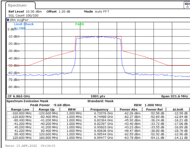
802.11ax (80MHz) / 6865MHz / Chain C / NSS-1
