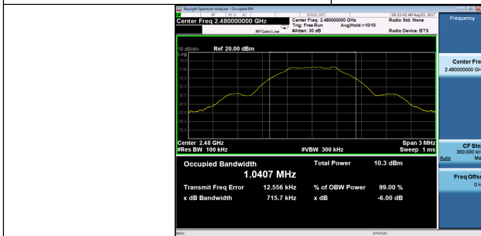
6dB BW –Bluetooth LE 2480MHz
