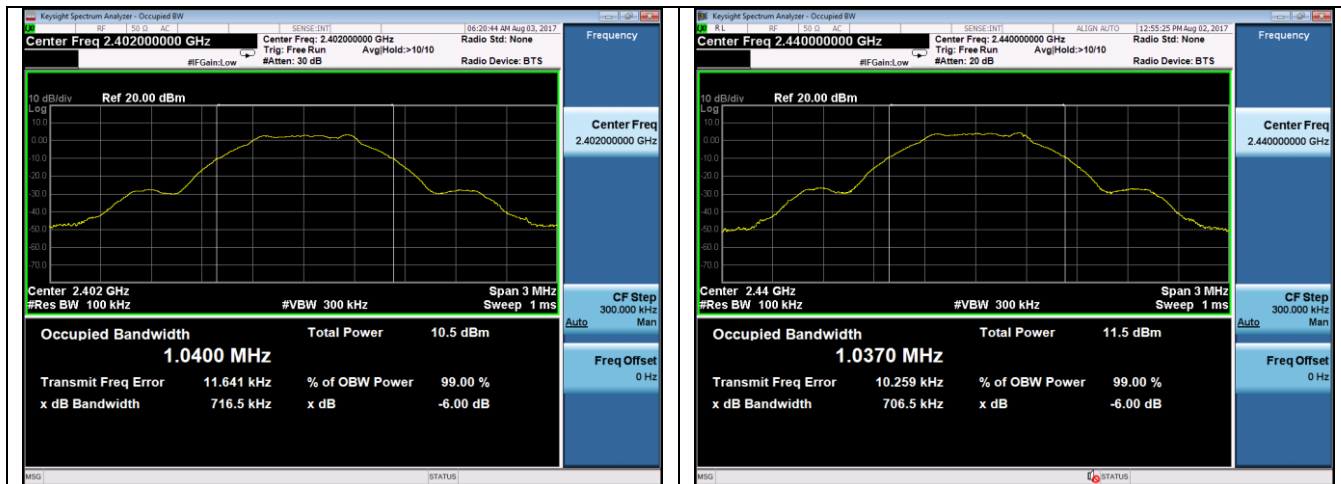
6dB BW –Bluetooth LE 2402MHz
