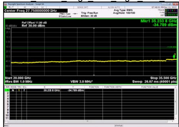
N77(15M)_DFT-s- OFDM QPSK Edge 1RB Right Low CH
