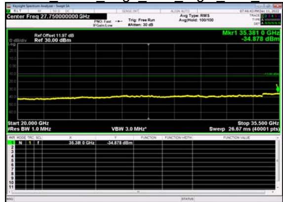
N77(15M)_DFT-s- OFDM BPSK Edge 1RB Right Low CH
