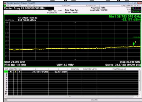
N77(90M)_DFT-s- OFDM BPSK Edge 1RB Left High CH
