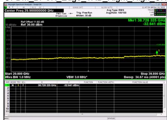
N77(90M)_DFT-s- OFDM BPSK Edge 1RB Right High CH
