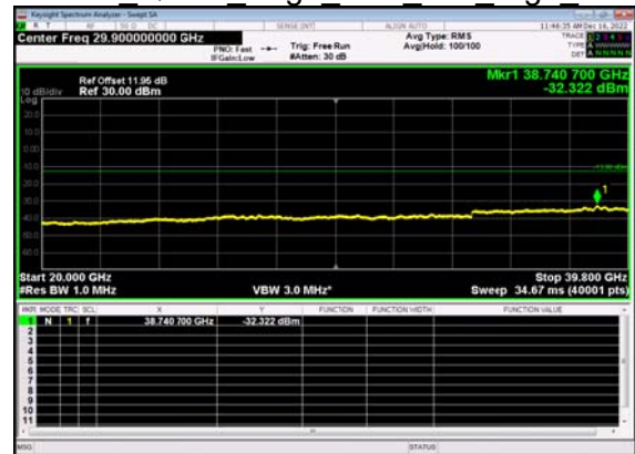
N77(90M)_DFT-s- OFDM QPSK Edge 1RB Left High CH
