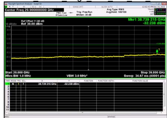
N77(100M)_DFT-s-OFDM QPSK Edge 1RB Left Mid CH
