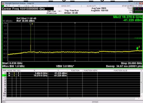
N77(15M)_DFT-s- OFDM QPSK Edge 1RB Right Low CH
