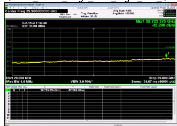
N77(100M)_DFT-s-OFDM BPSK Edge 1RB Right Mid CH
