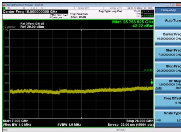
U-NII-2a ,Plot 4,7000MHz~26000MHz-802 .11ac(20MHz),5260MHz
