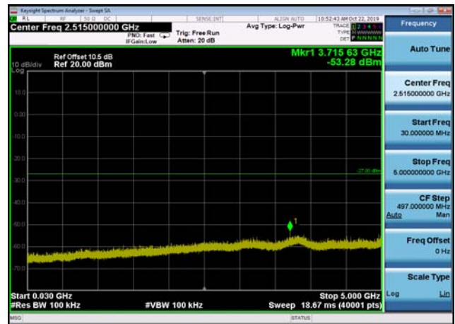
U-NII-2a ,Plot 2,30MHz~5000MHz-802.11 ac(80MHz),5290MHz
