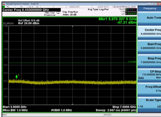
U-NII-2a ,Plot 3,5900MHz~7000MHz-802. 11ac(20MHz),5300MHz
