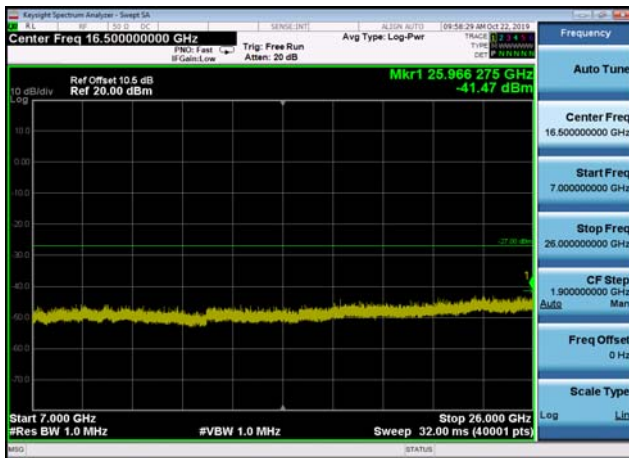
U-NII-2a ,Plot 4,7000MHz~26000MHz-802 .11ac(40MHz),5310MHz
