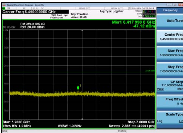
U-NII-2c ,Plot 3,5900MHz~7000MHz-802. 11a(20MHz),5700MHz
