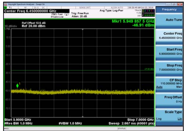
U-NII-2a ,Plot 3,5900MHz~7000MHz-802. 11ac(20MHz),5320MHz
