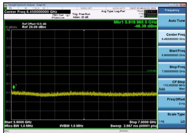
U-NII-2a ,Plot 3,5900MHz~7000MHz-802. 11ac(40MHz),5310MHz
