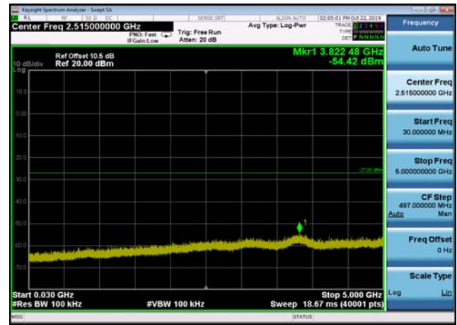
U-NII-2c ,Plot 2,30MHz~5000MHz-802.11 a(20MHz),5700MHz
