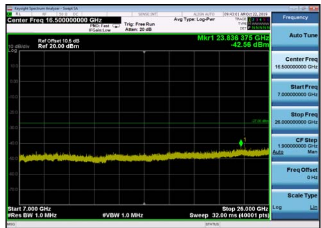
U-NII-2a ,Plot 4,7000MHz~26000MHz-802 .11ac(20MHz),5300MHz
