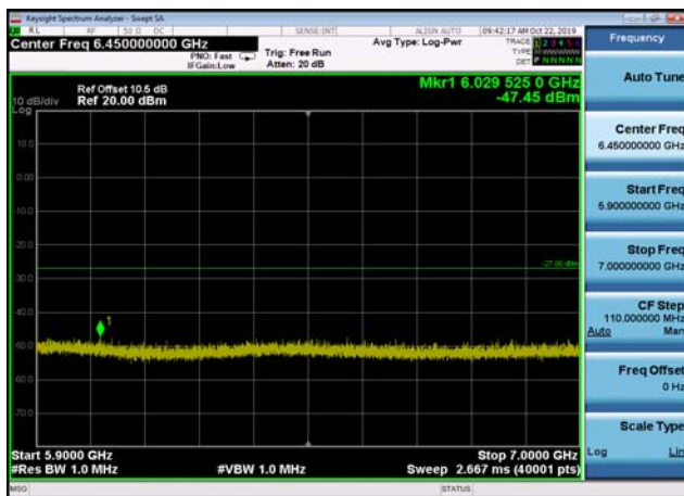
U-NII-2a ,Plot 3,5900MHz~7000MHz-802. 11ac(40MHz),5270MHz
