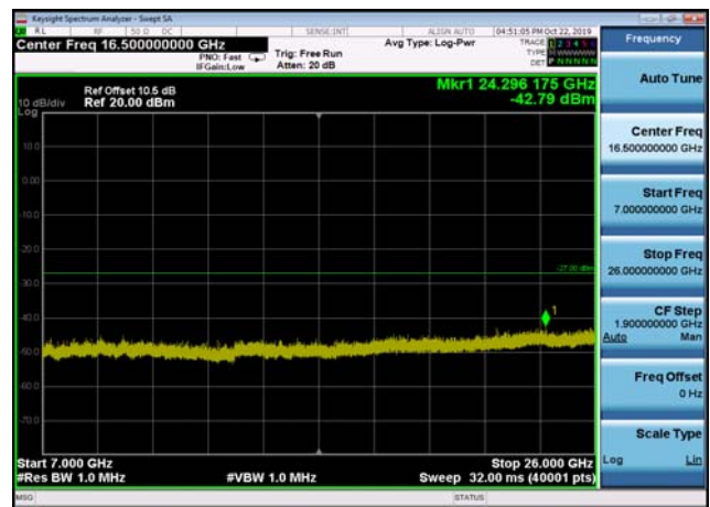
U-NII-2c ,Plot 4,7000MHz~26000MHz-802 .11ac(40MHz),5670MHz
