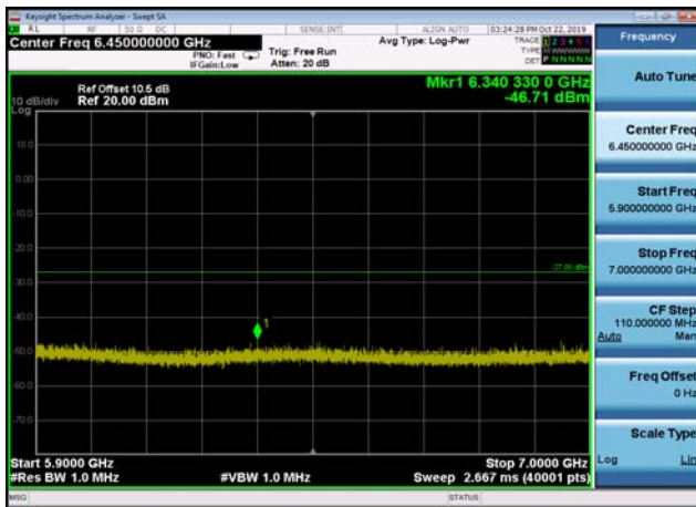
U-NII-2c ,Plot 3,5900MHz~7000MHz-802. 11ac(40MHz),5510MHz
