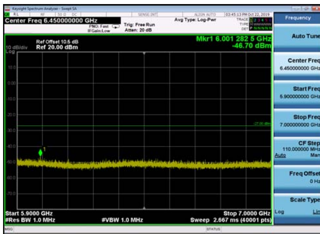
U-NII-2c ,Plot 3,5900MHz~7000MHz-802.11n(40MHz),5510MHz
