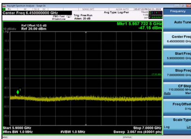
U-NII-2a ,Plot 3,5900MHz~7000MHz-802. 11a(20MHz),5260MHz
