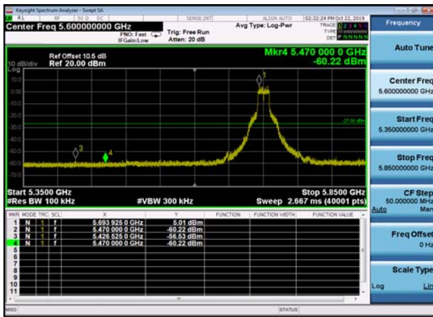
U-NII-2c ,Plot 1,Band Edge-802.11ac(20 MHz),5600MHz
