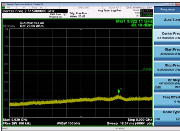
U-NII-2a ,Plot 2,30MHz~5000MHz-802.11 ac(40MHz),5310MHz
