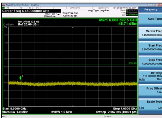
U-NII-2c ,Plot 3,5900MHz~7000MHz-802. 11ac(40MHz),5670MHz
