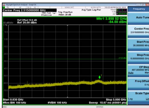
U-NII-2c ,Plot 2,30MHz~5000MHz-802.11 ac(40MHz),5510MHz
