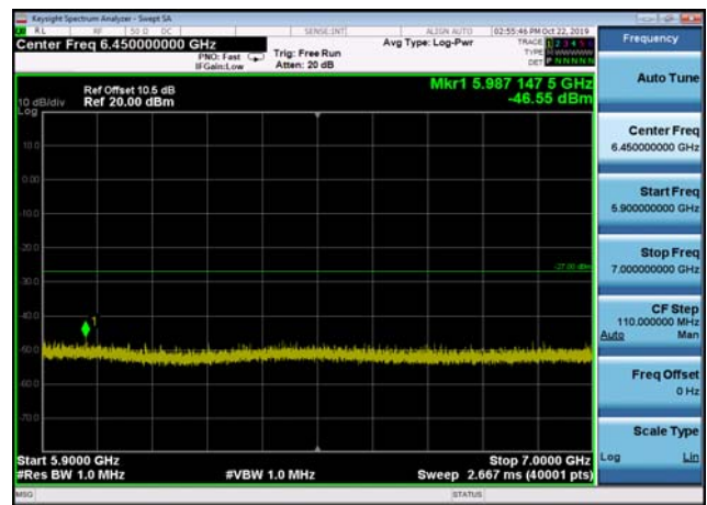
U-NII-2c ,Plot 3,5900MHz~7000MHz-802.11n(20MHz),5600MHz
