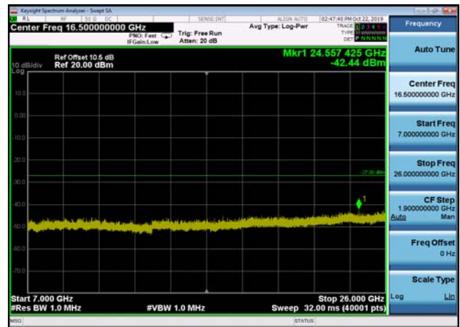
U-NII-2c ,Plot 4,7000MHz~26000MHz-802 .11n(20MHz),5700MHz
