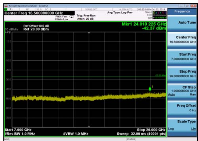
U-NII-2c ,Plot 4,7000MHz~26000MHz-802 .11ac(20MHz),5600MHz
