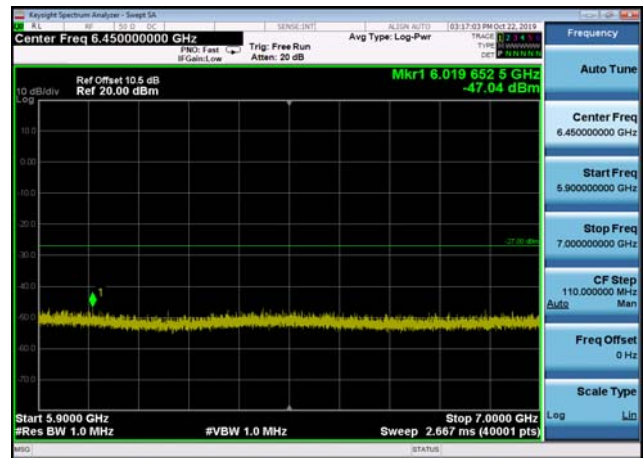
U-NII-2c ,Plot 3,5900MHz~7000MHz-802. 11ac(40MHz),5590MHz
