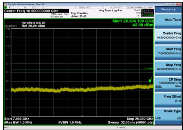
U-NII-2c ,Plot 4,7000MHz~26000MHz-802 .11a(20MHz),5700MHz
