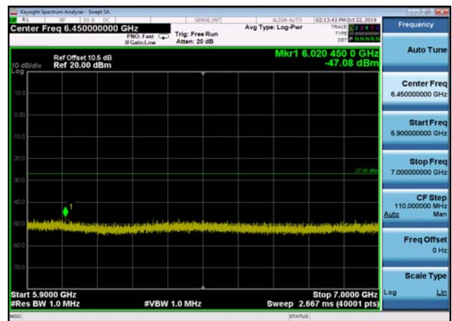
U-NII-2c ,Plot 3,5900MHz~7000MHz-802. 11ac(20MHz),5500MHz
