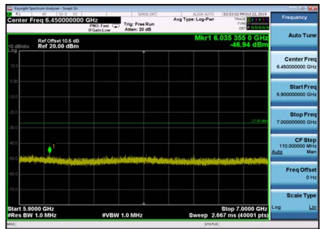
U-NII-2c ,Plot 3,5900MHz~7000MHz-802.11n(40MHz),5590MHz
