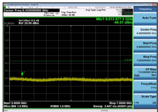
U-NII-2c ,Plot 3,5900MHz~7000MHz-802. 11ac(80MHz),5530MHz
