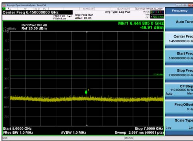
U-NII-2c ,Plot 3,5900MHz~7000MHz-802.11n(20MHz),5500MHz
