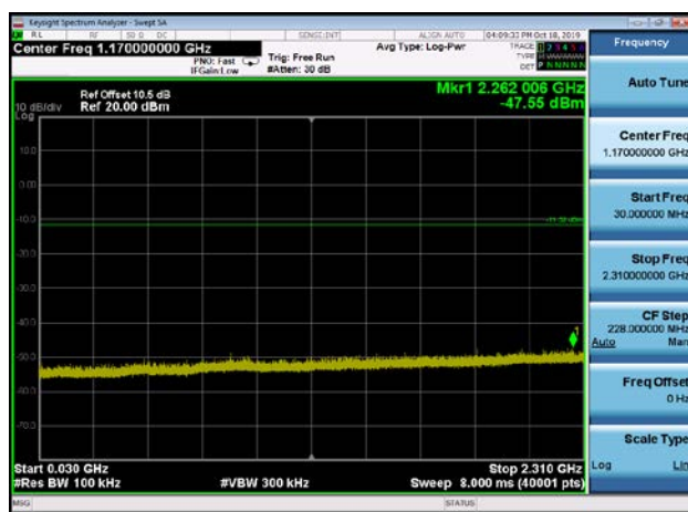
,Plot 3,30MHz~2310MHz-802.11b,2462MHz
