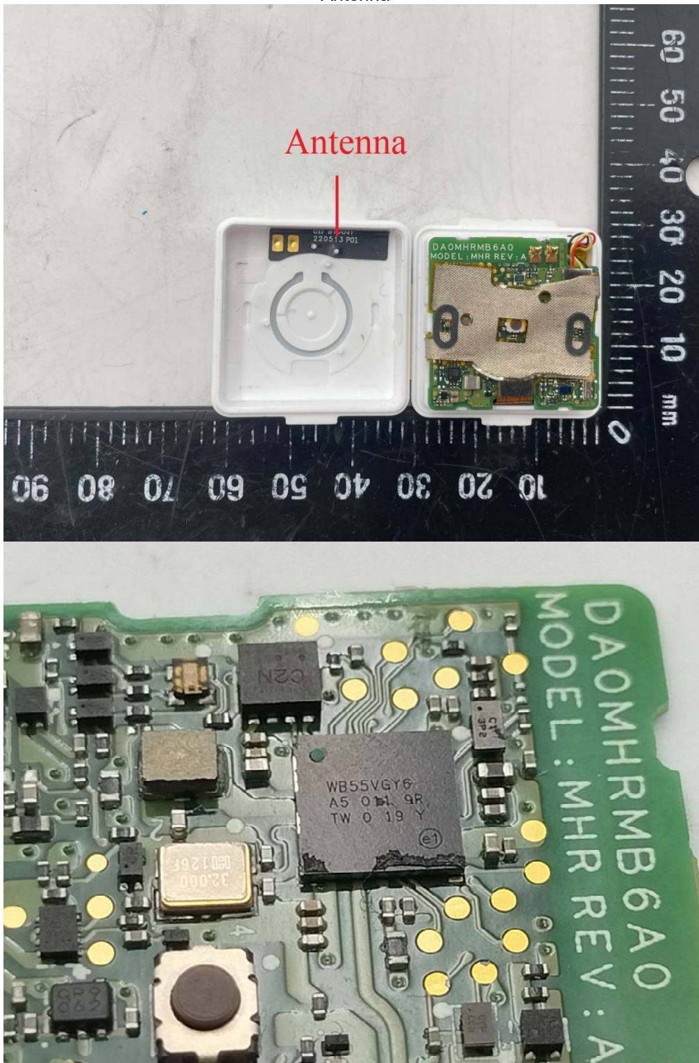
Antenna
