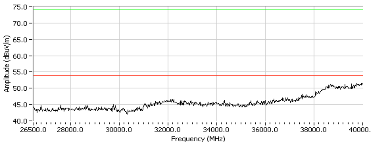
5785MHz, Chain A, 802.11n-20
