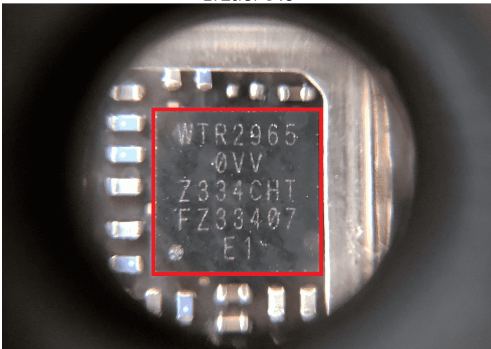
WiFi&amp;BT IC
