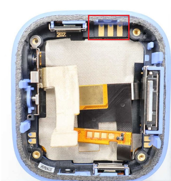
LTE Antenna
