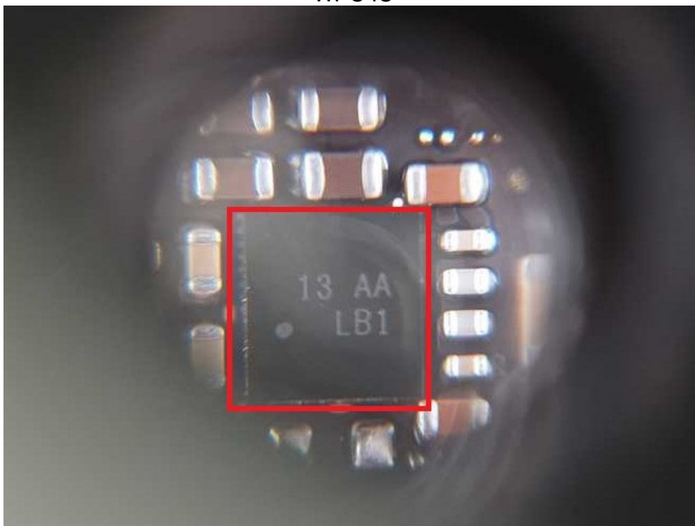
WPC IC
