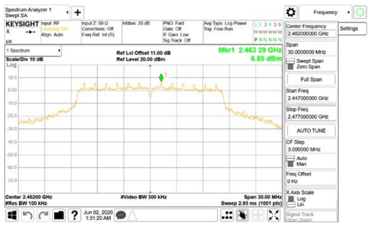
FCC_15_247_WLAN\Reference Level_802.11g_20MHz_Chain0_2462MHz
